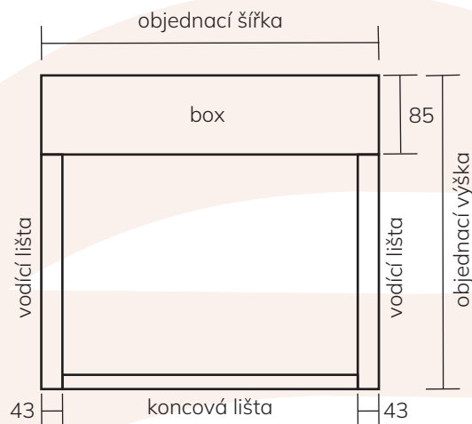
ČELNÍ POHLED Z EXTERIÉRU
