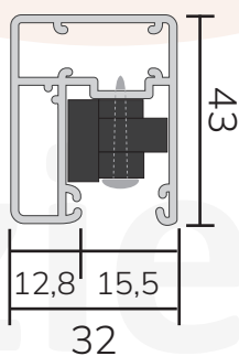
VODÍCÍ LIŠTA S OSAZENÝM KLIK-KLAK SYSTÉMEM
