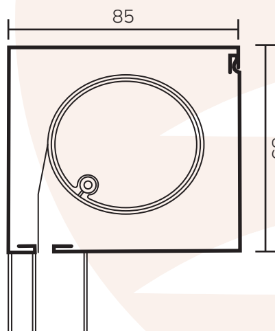
ŘEZ NAVÍJECÍM BUBNEM
